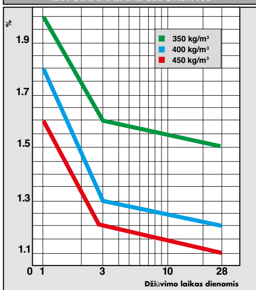
LIEKAMOJI DRĒGMĒ MAPECEM IŠLYGINAMAJAME SLUOKSNYJE
