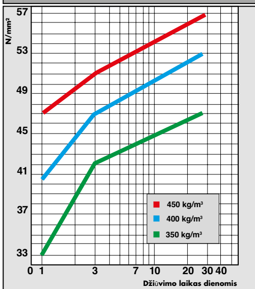
MAPECEM GNIUŽDOMASIS STĪPRIS NAUDOJANT SKIRTINGUS MIŠINIUS
