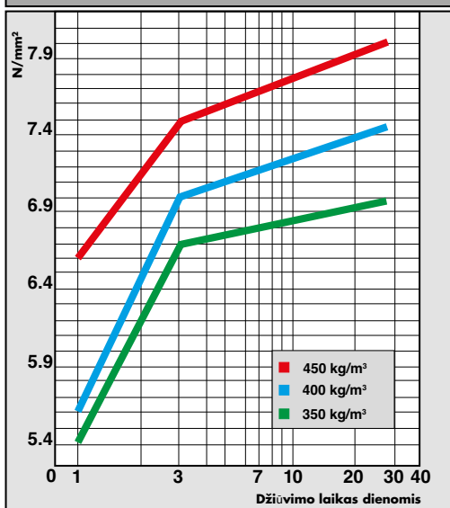
MAPECEM LENKIAMASIS STĪPRIS NAUDOJANT SKIRTINGUS MIŠINIUS
